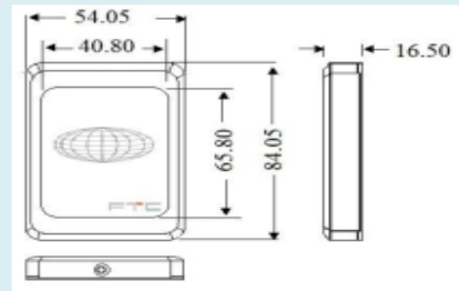
设备尺寸图
